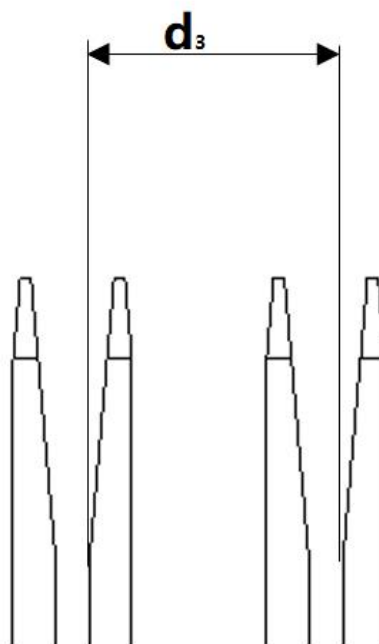
图7 相邻两片顶齿片间距测量示意图
