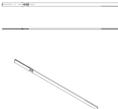
图4 顶齿片结构示例
